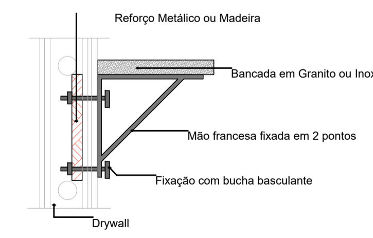
DET REFORÇO DRYWALL
